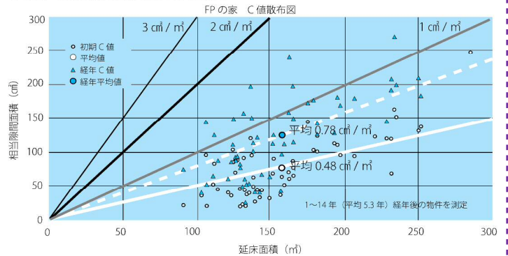
「FPの家」の気密性能【初期値と経年後の実測値】
